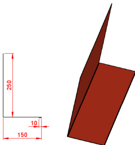
Liitoslista LL-411 (3000 mm x 0,5 mm) OVH 29,07 € sis. alv 23 %
