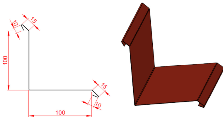
Sisäkulmalista SKL-252 (3000 mm x 0,5 mm) OVH 23,68 € sis. alv 23 %
