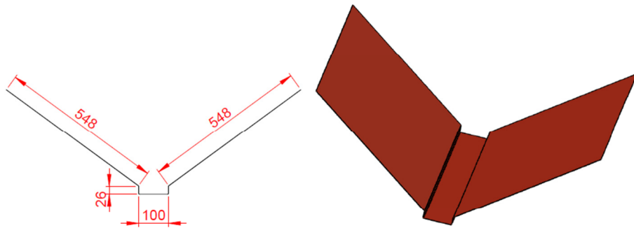
Sisäjiirilista SJL-1250 (3000 mm x 0,6 mm) OVH 79,33 € sis. alv 23 %
