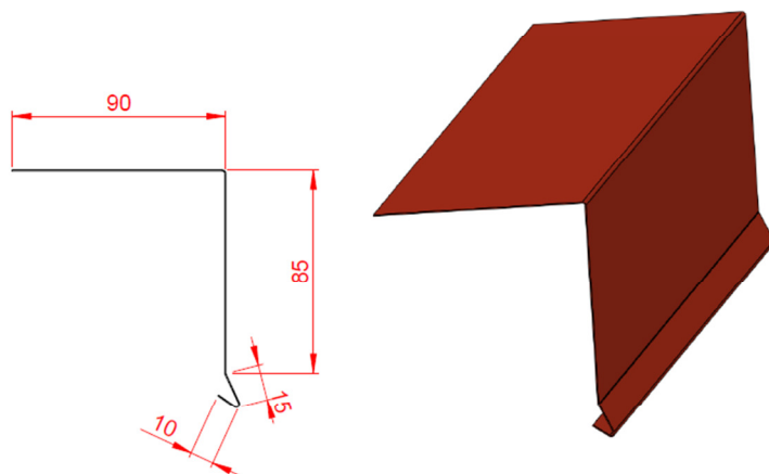
Alaräystäslista ARL-200 (3000 mm x 0,5 mm) OVH 18,22 sis. alv 23 %
