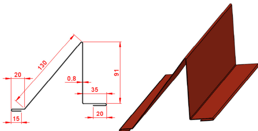
Lumiestelista LEL-313 (3000 mm x 0,6 mm) OVH 25,46 € sis. alv 23 %
